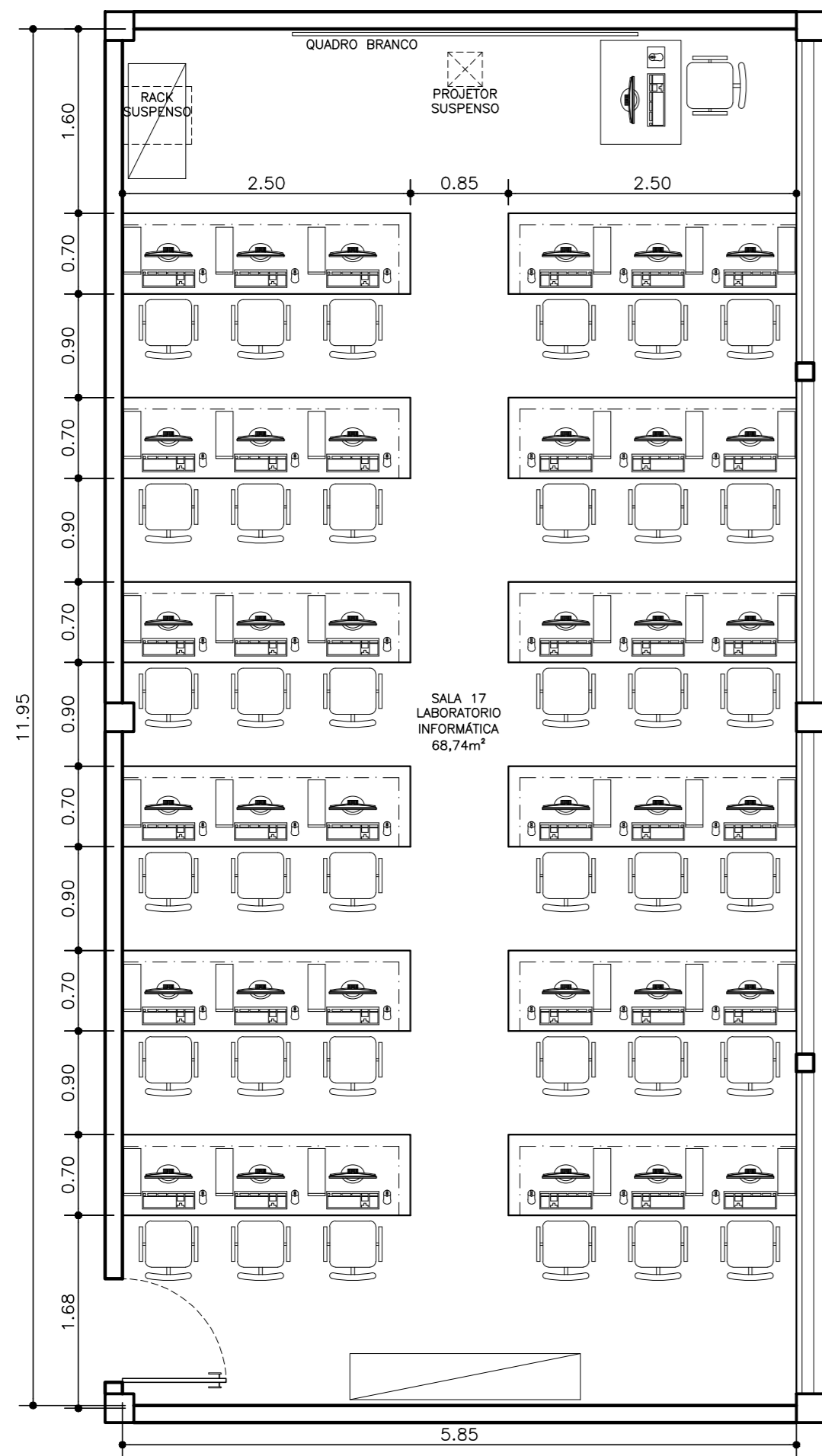
PLANTA BAIXA - LAYOUT
