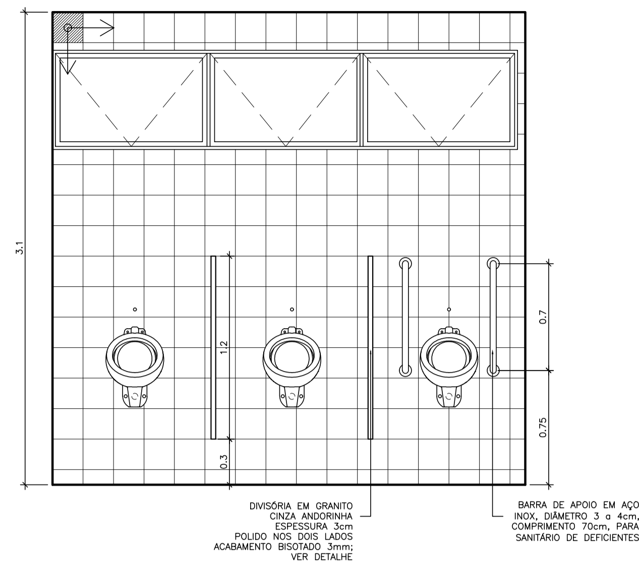
VISTA D ESCALA 1:25
