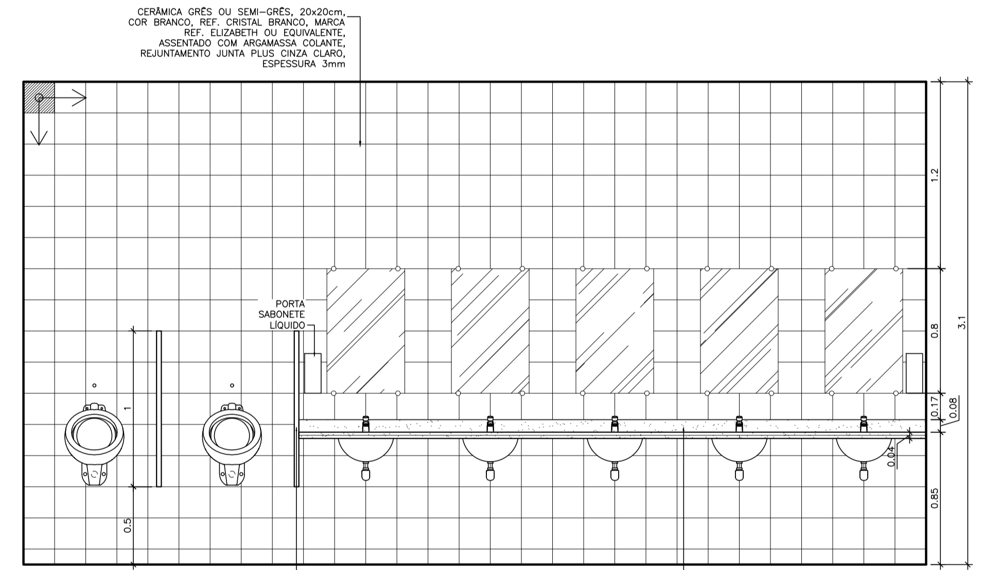
VISTA C ESCALA 1:25
