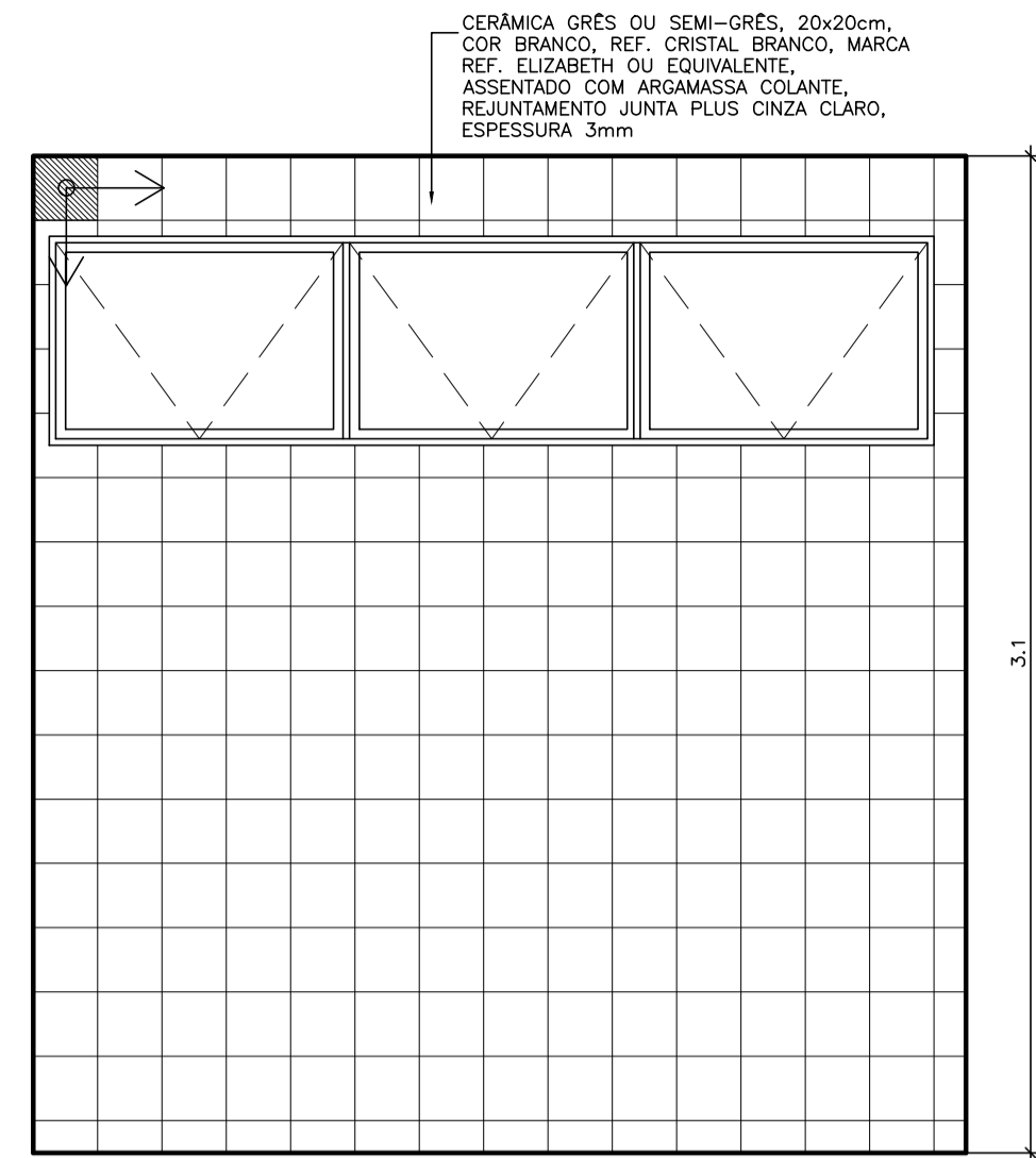
VISTA D ESCALA 1:25
