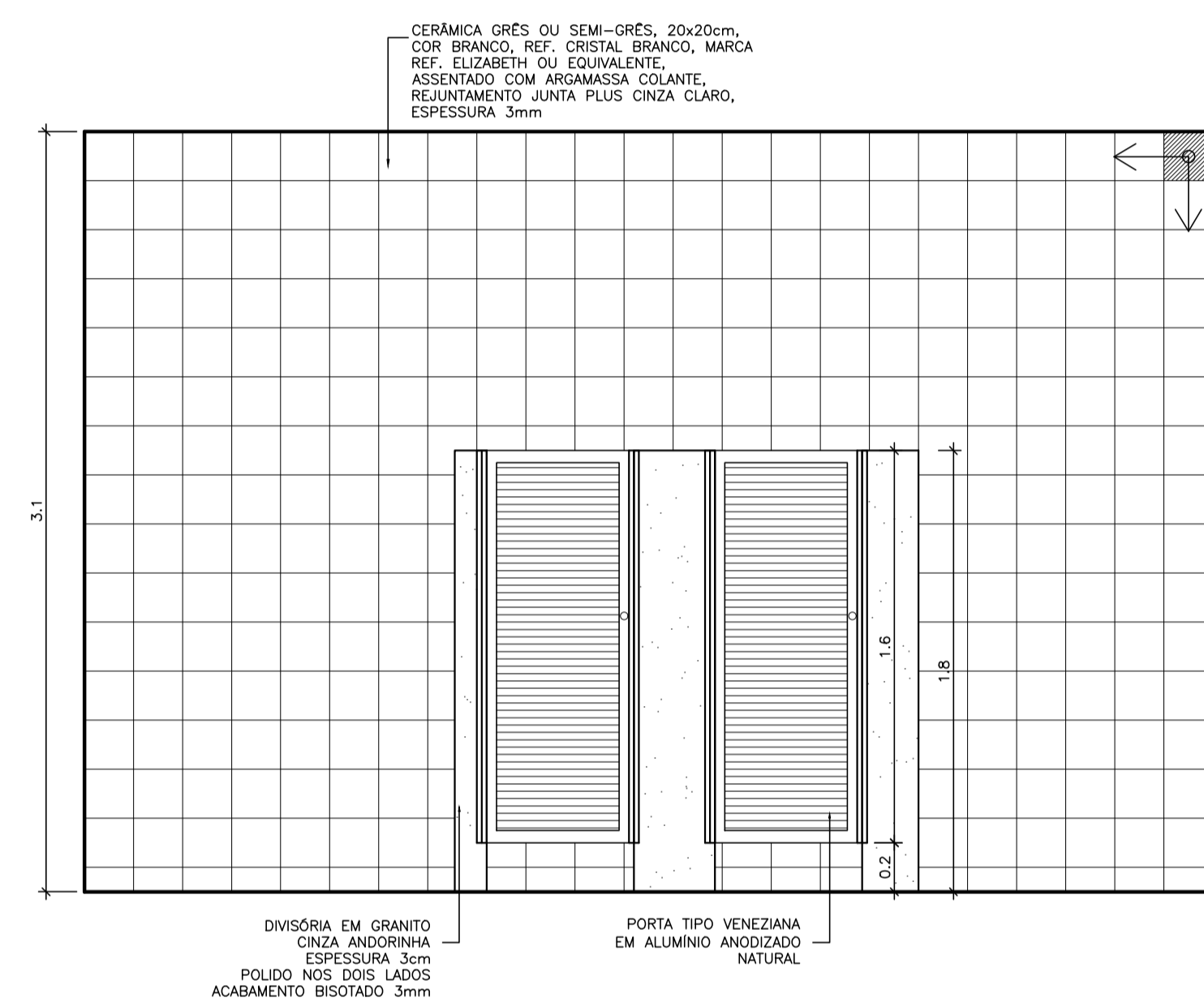
VISTA A ESCALA 1:25
