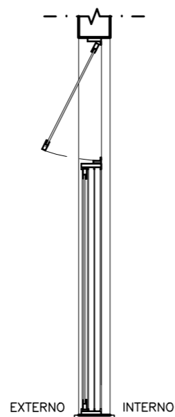
CORTE - J3
