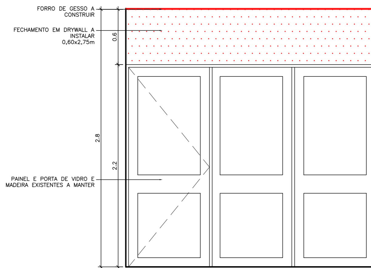
VISTA 2 ESCALA 1:25
