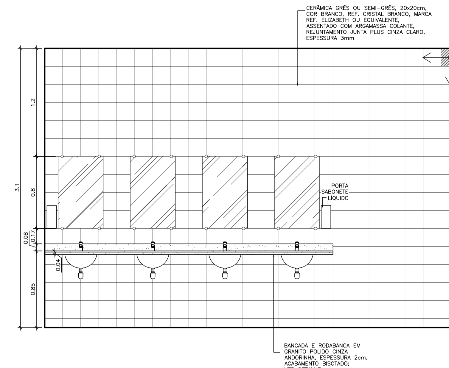
VISTA C ESCALA 1:25
