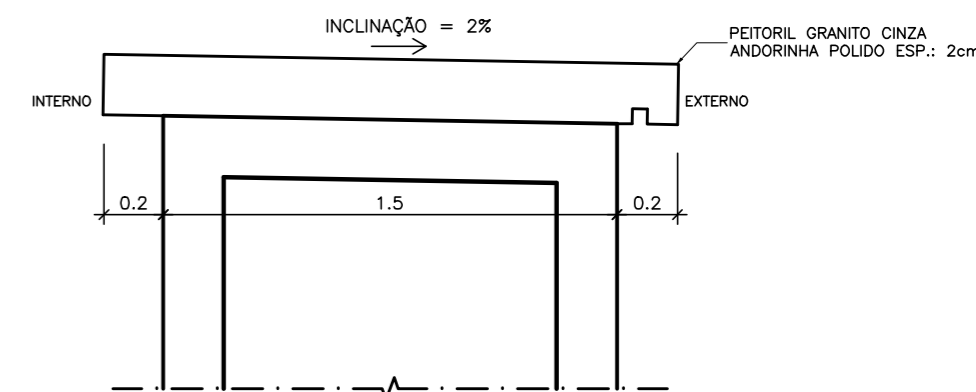
DETALHE PEITORIL
