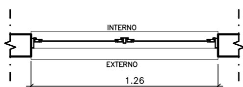
PLANTA BAIXA - J2
