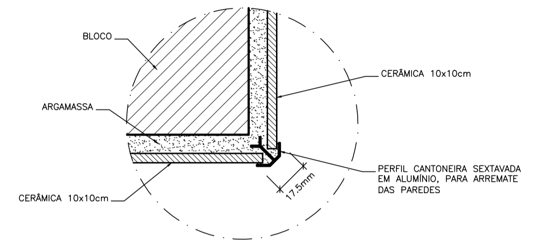
DETALHE PERFIL DE CANTO SEM ESCALA
