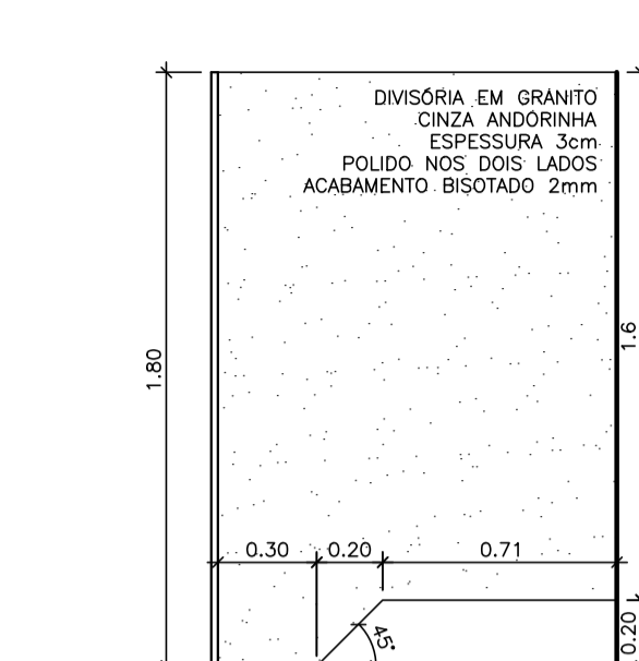
DET. DIVISÓRIA SANITÁRIOS ESCALA 1:25
