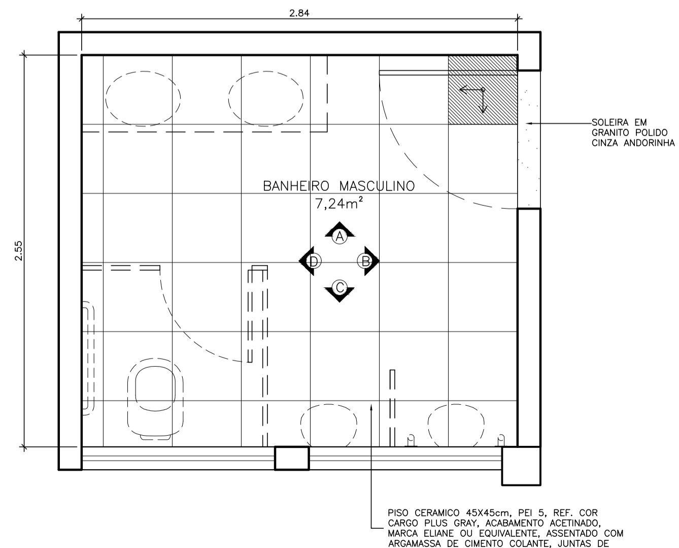
PAGINAÇÃO DE PISO ESCALA 1:25
