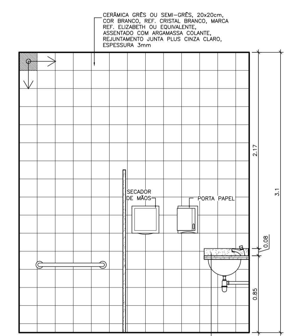
VISTA D ESCALA 1:25
