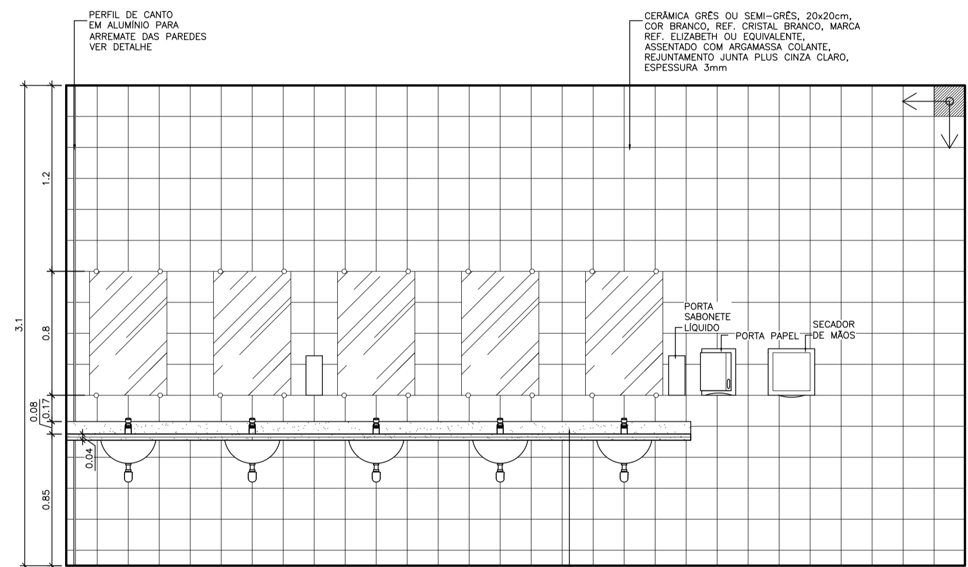
VISTA C ESCALA 1:25
