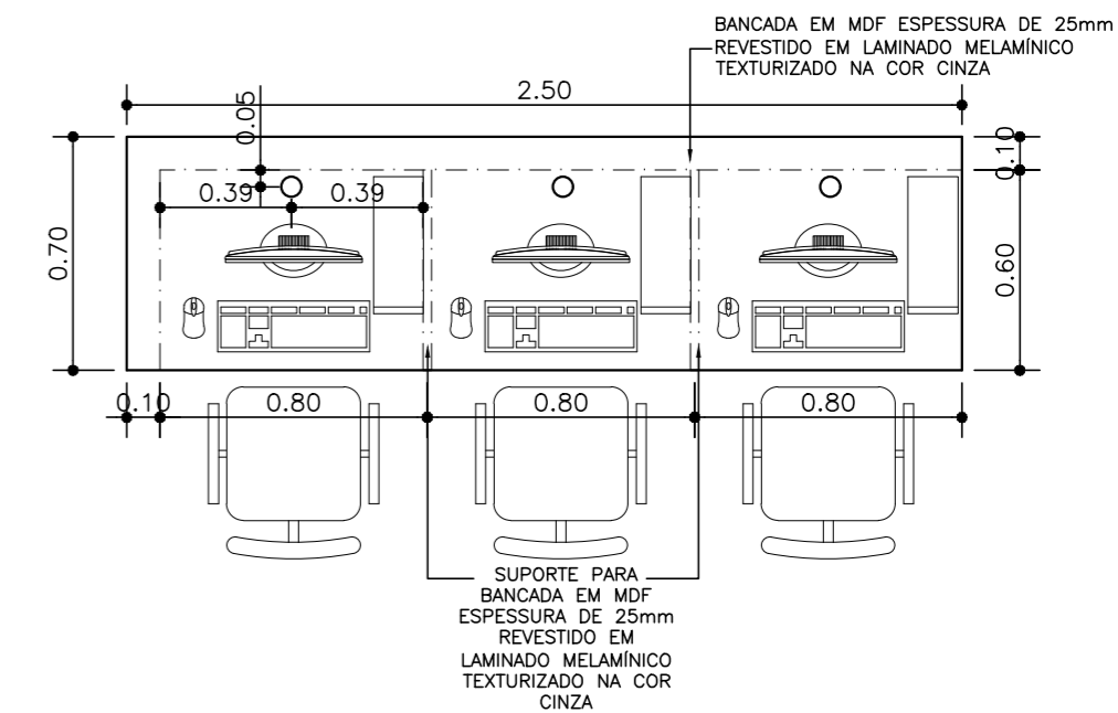
DET. BANCADA - PLANTA BAIXA
