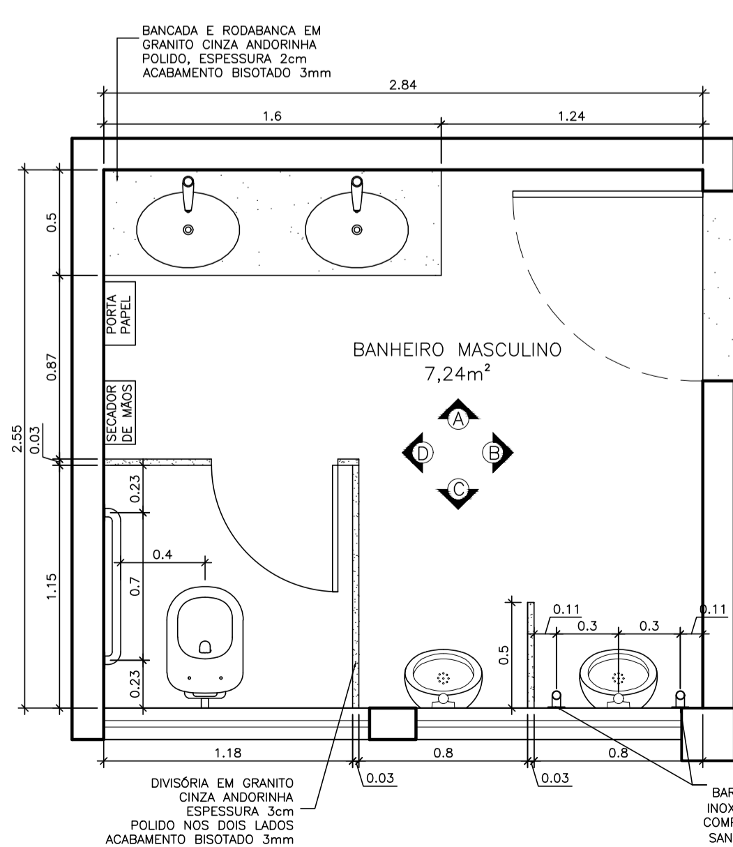
PLANTA BAIXA BANHEIRO MASC. ESCALA 1:25
