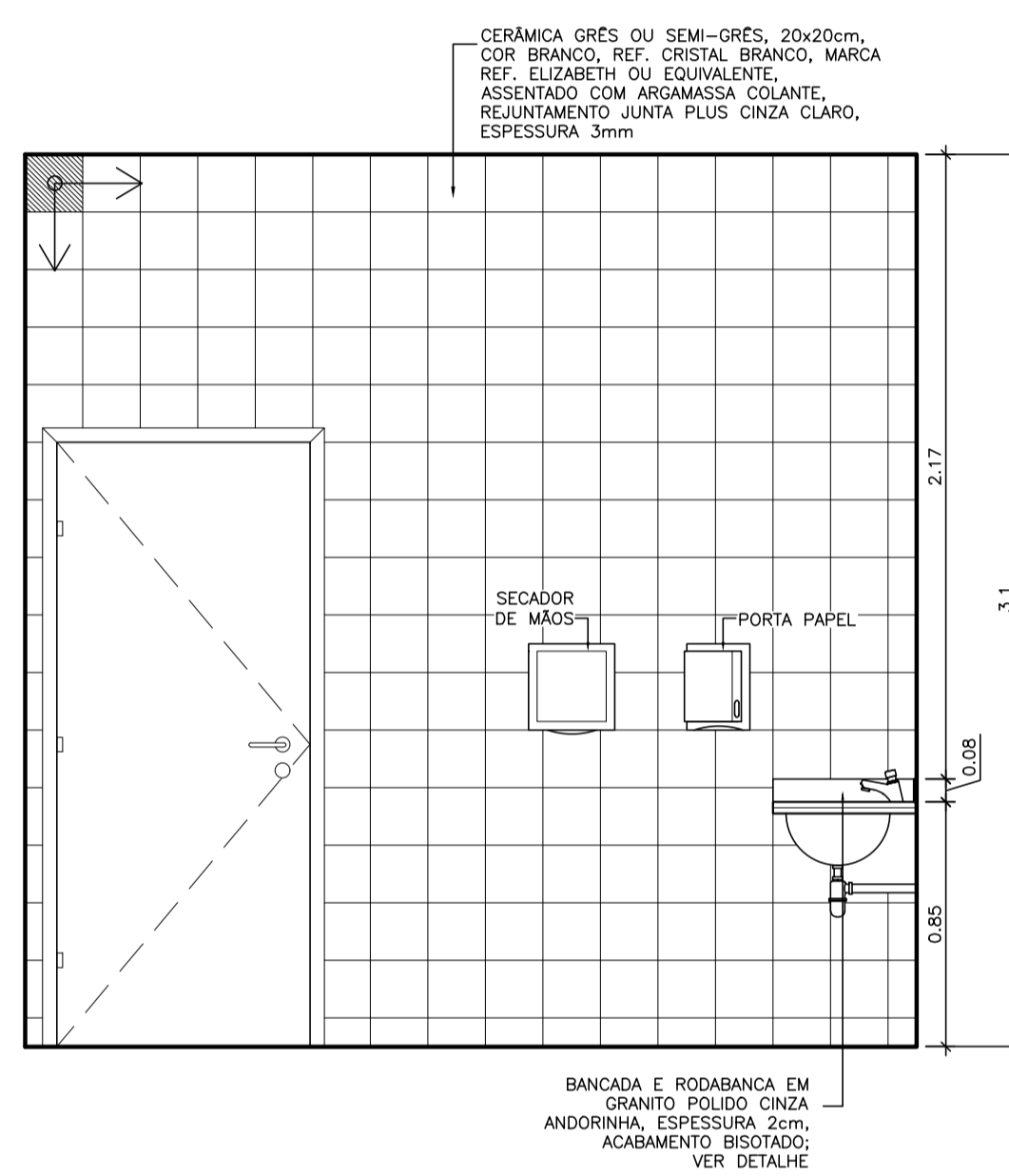
VISTA B ESCALA 1:25
