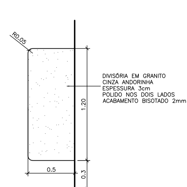
DET. DIVISÓRIA MICTÓRIOS ESCALA 1:25
