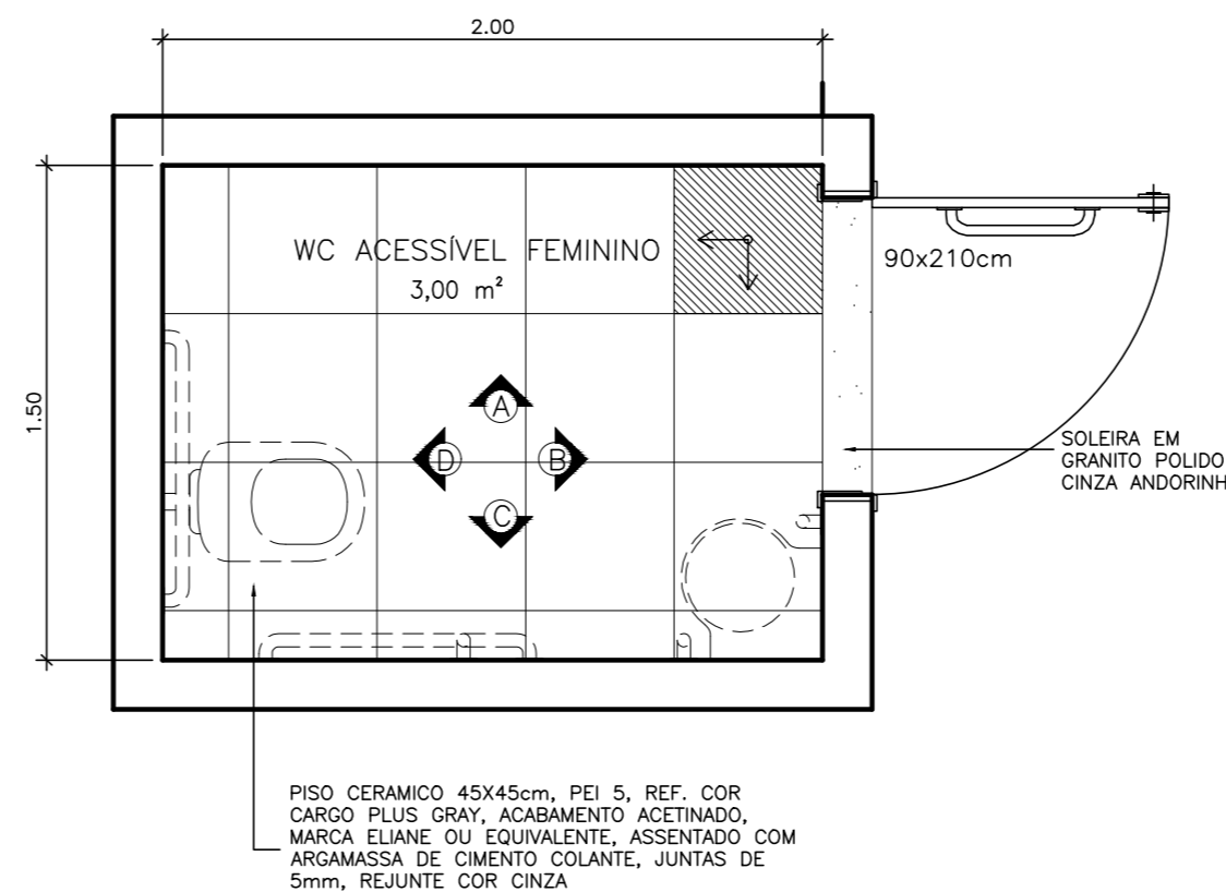
PAGINAÇÃO DE PISO ESCALA 1:25
