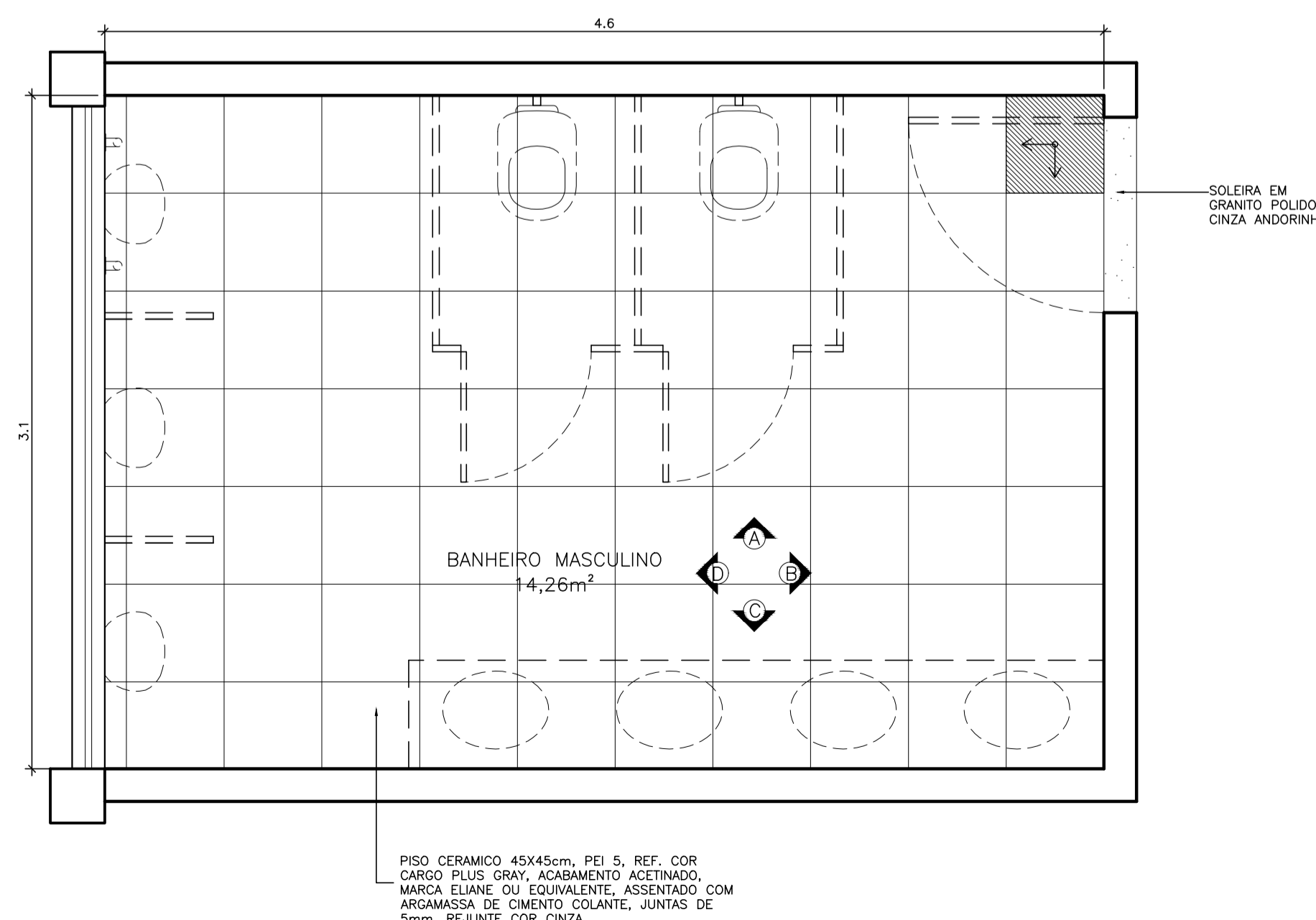
PAGINAÇÃO DE PISO ESCALA 1:25
