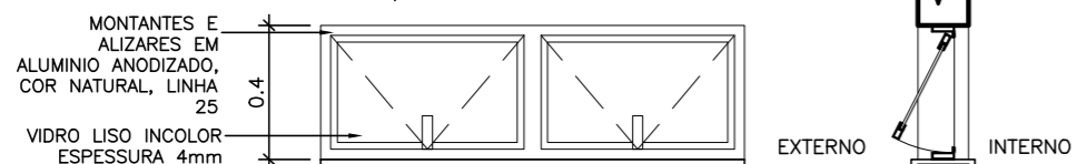
VISTA - J2
