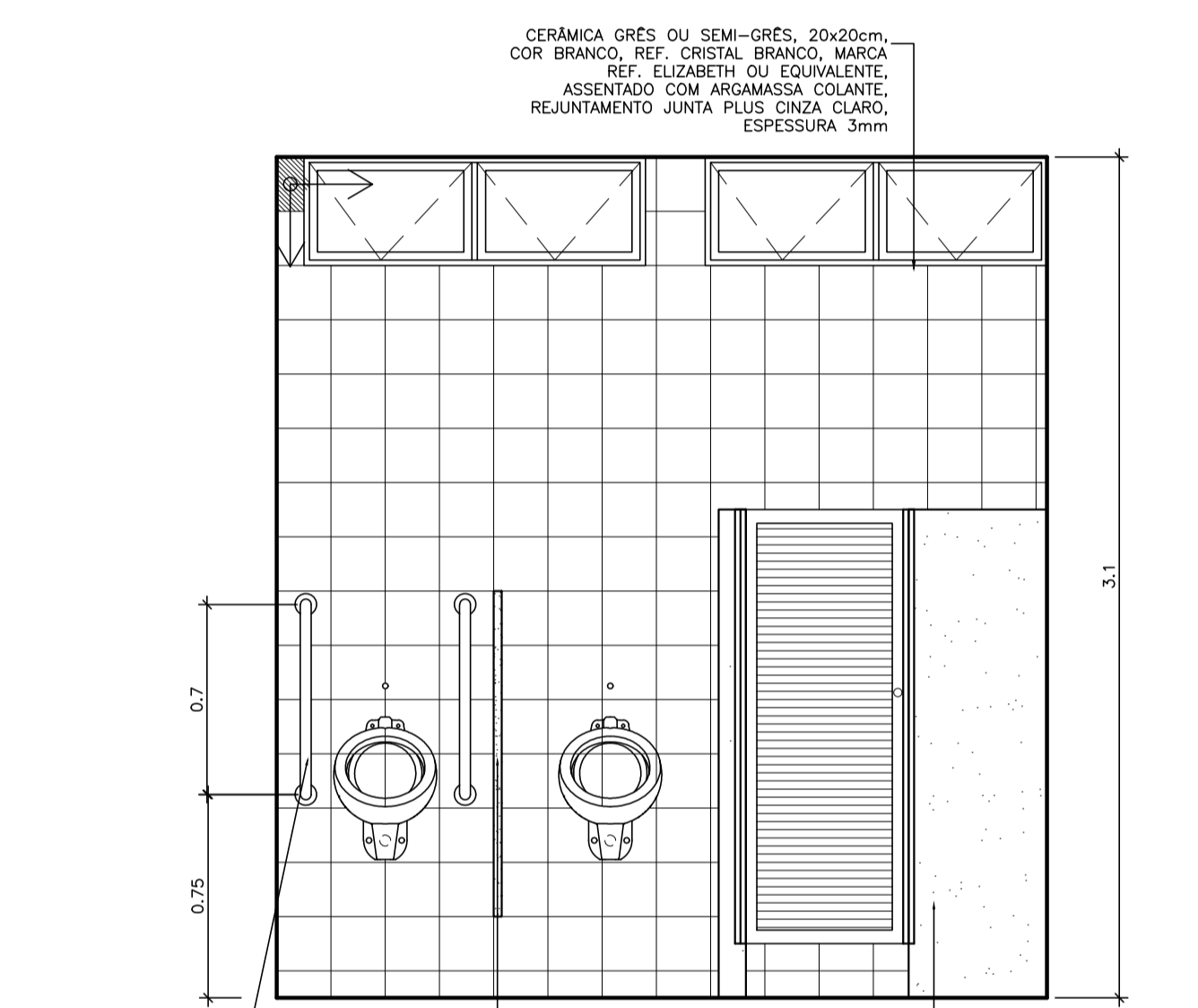
VISTA C ESCALA 1:25
