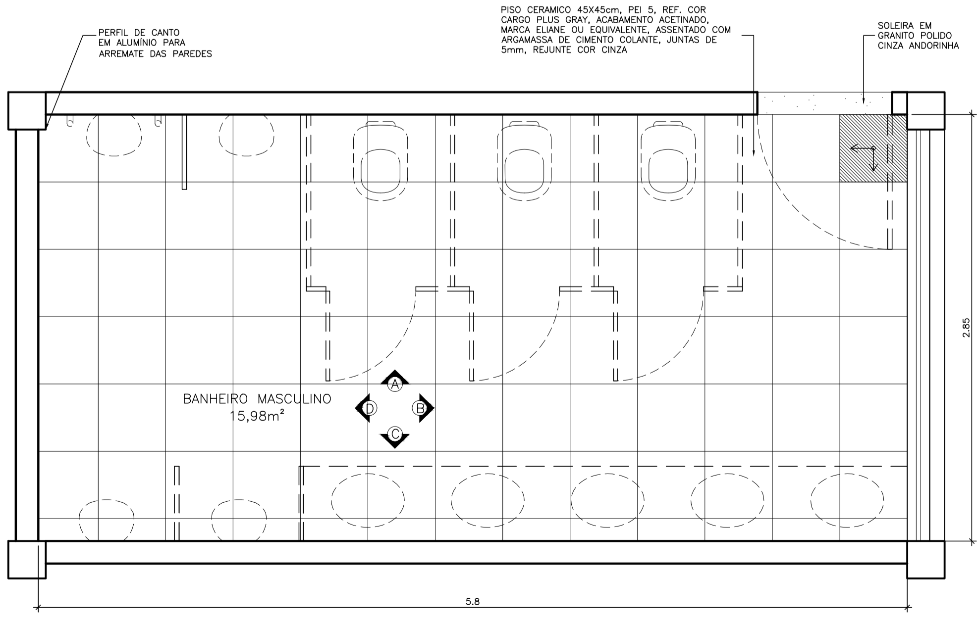
PAGINAÇÃO DE PISO ESCALA 1:25
