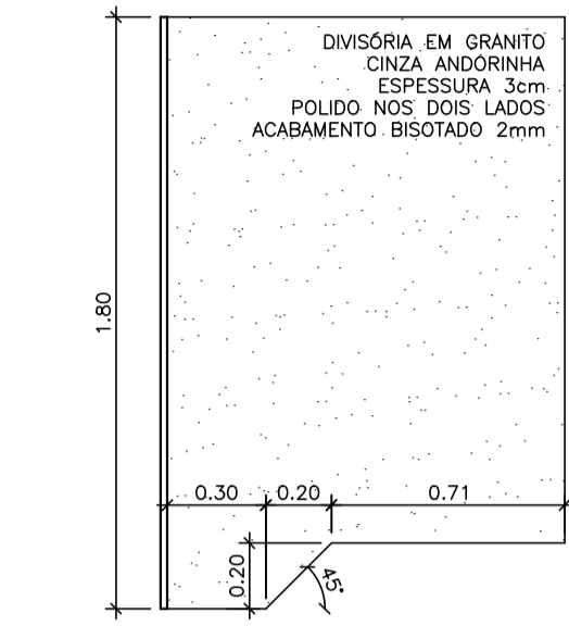
DET. DIVISÓRIA SANITÁRIOS ESCALA 1:25
