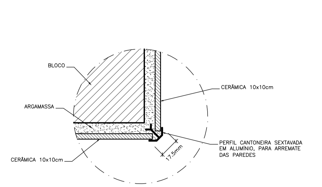
DETALHE PERFIL DE CANTO SEM ESCALA
