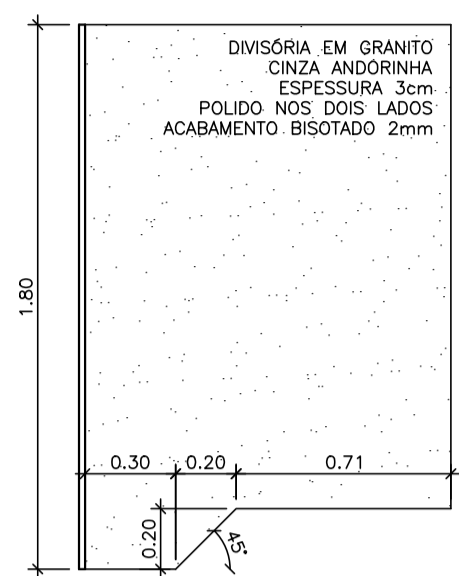
DET. DIVISÓRIA SANITÁRIOS ESCALA 1:25
