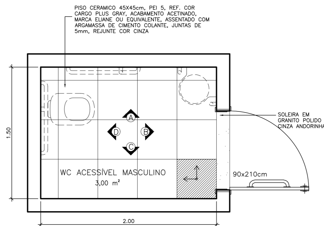
PAGINAÇÃO DE PISO ESCALA 1:25
