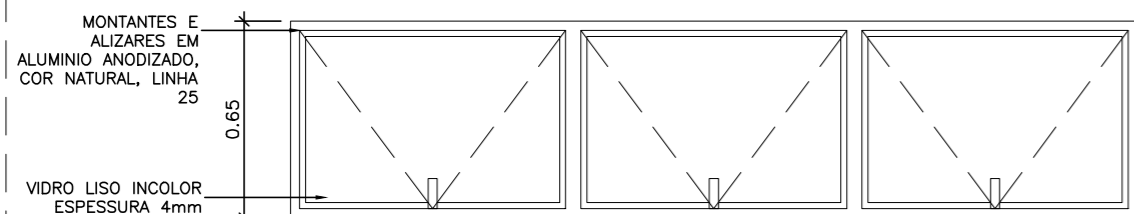
VISTA - J1
