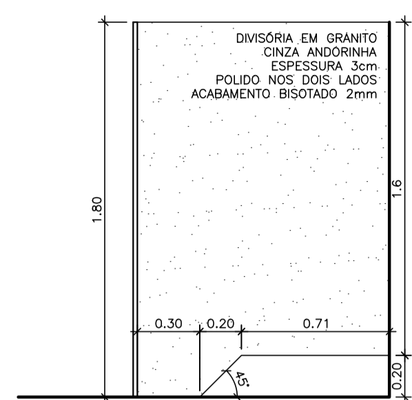
DET. DIVISÓRIA SANITÁRIOS ESCALA 1:25
