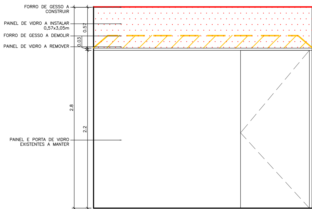
VISTA 1 ESCALA 1:25
