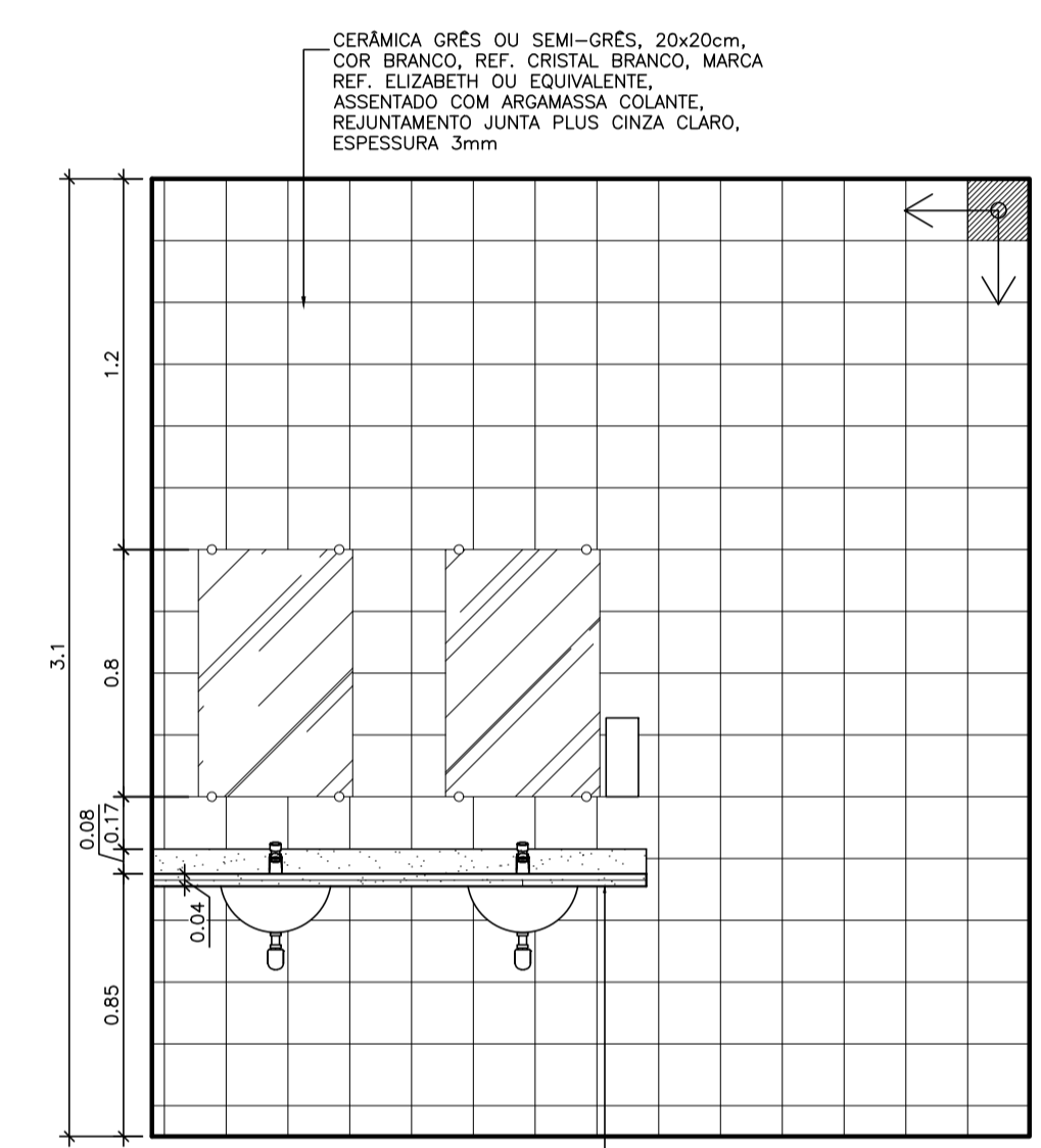
VISTA A ESCALA 1:25
