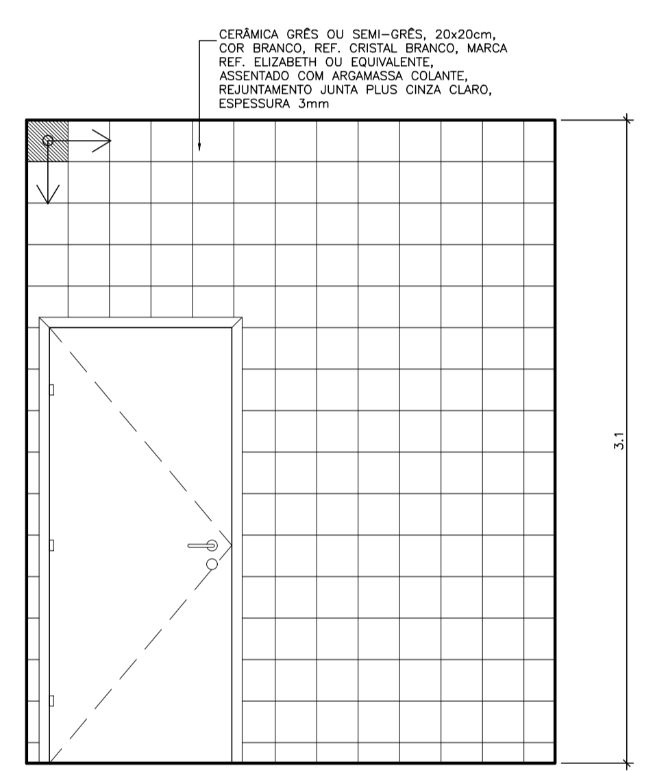
VISTA B ESCALA 1:25
