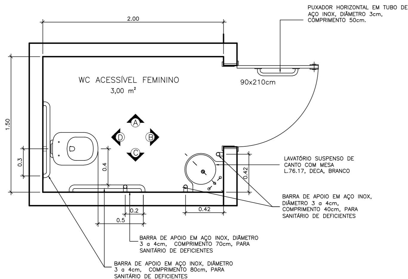
PLANTA BAIXA WC ACESS. FEM. ESCALA 1:25
