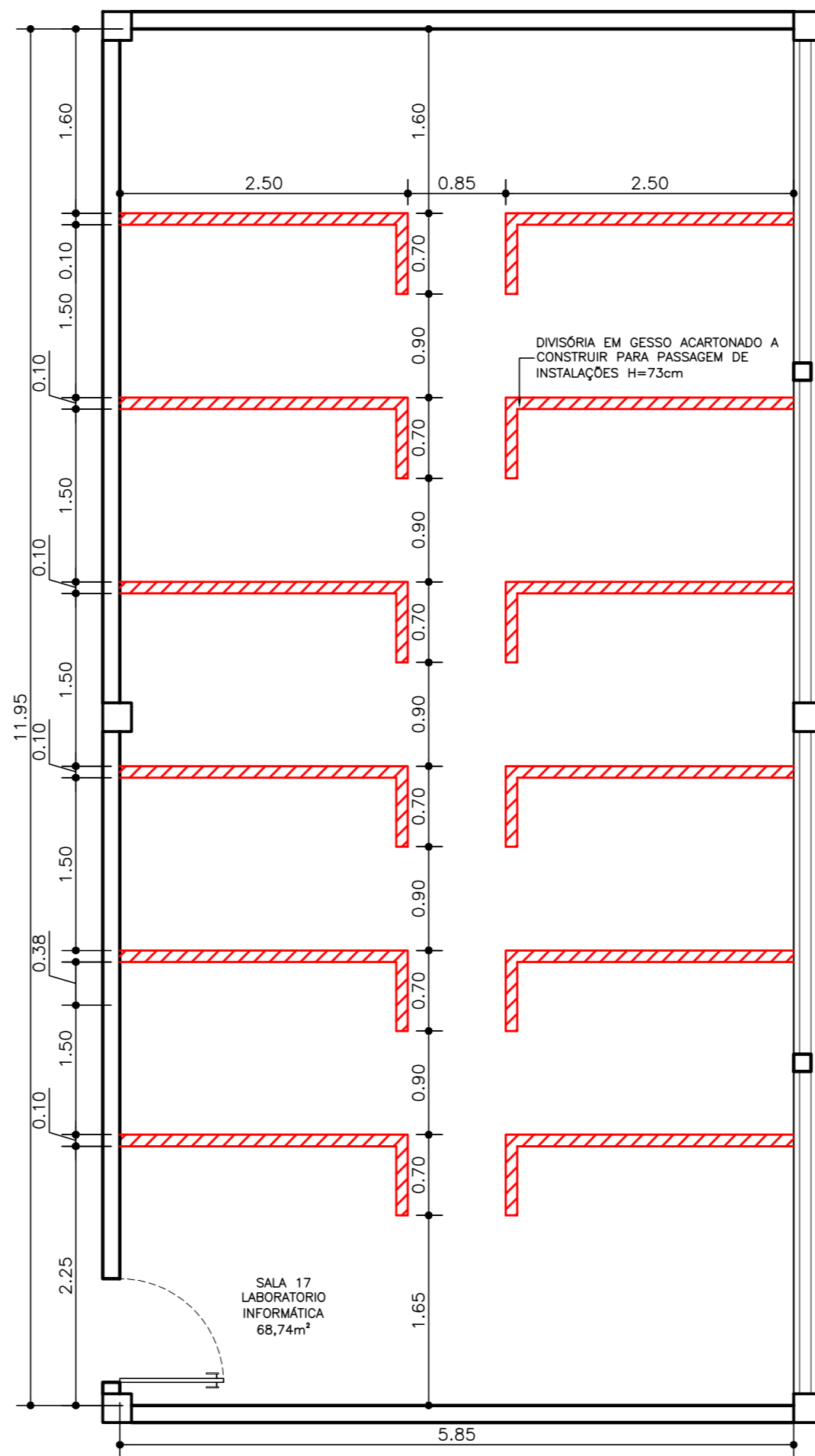
PLANTA BAIXA - A CONSTRUIR
