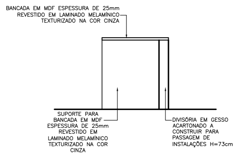
DET. BANCADA - CORTE
