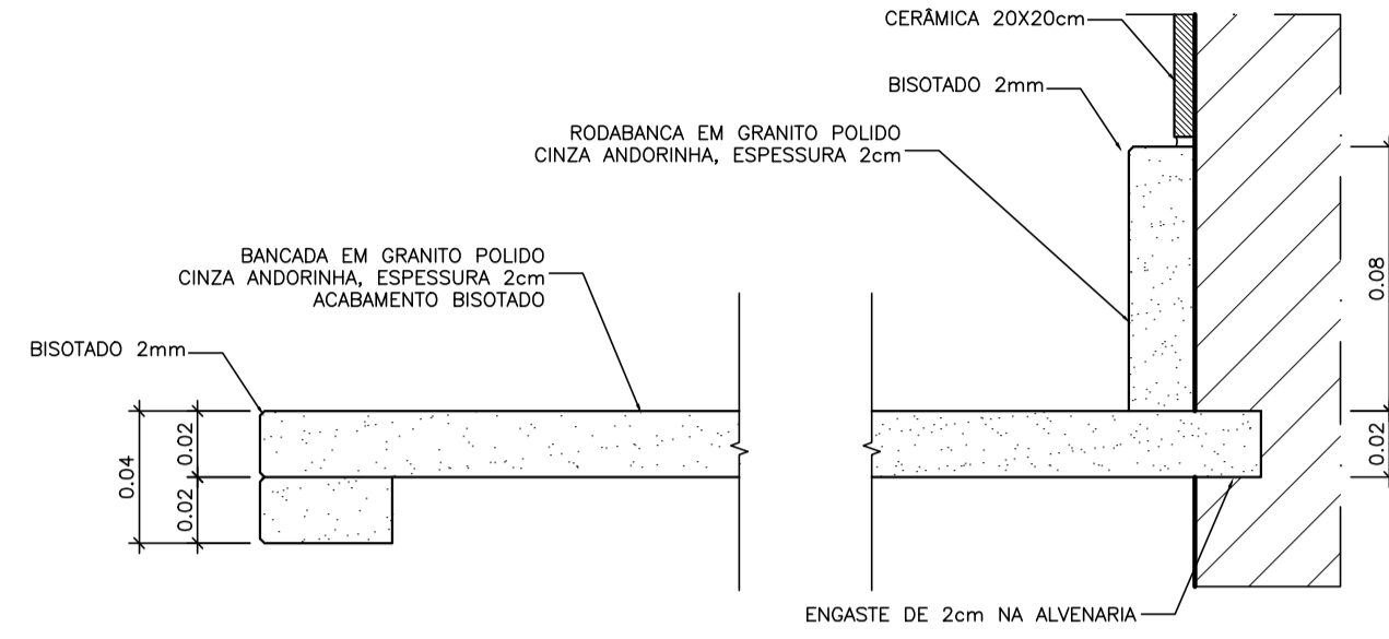
DETALHE BORDA E RODABANCA DA BANCADA ESCALA 1:2.5
