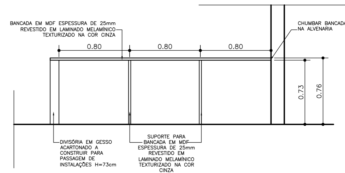
DET. BANCADA - VISTA
