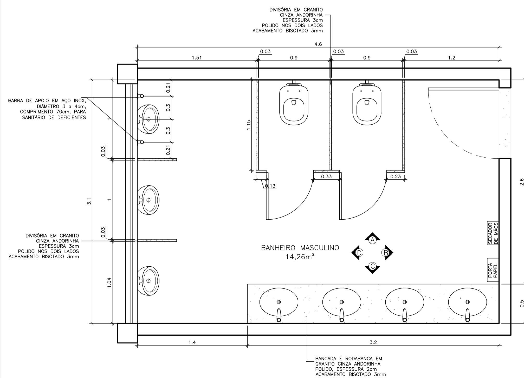
PLANTA BAIXA BANHEIRO MASC. ESCALA 1:25
