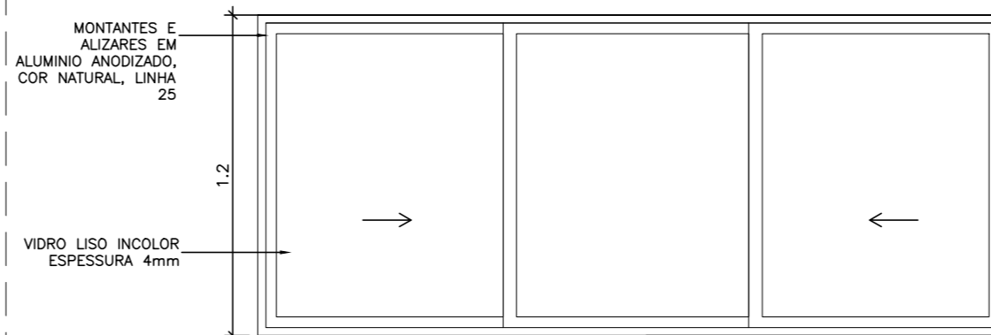
VISTA - J4
