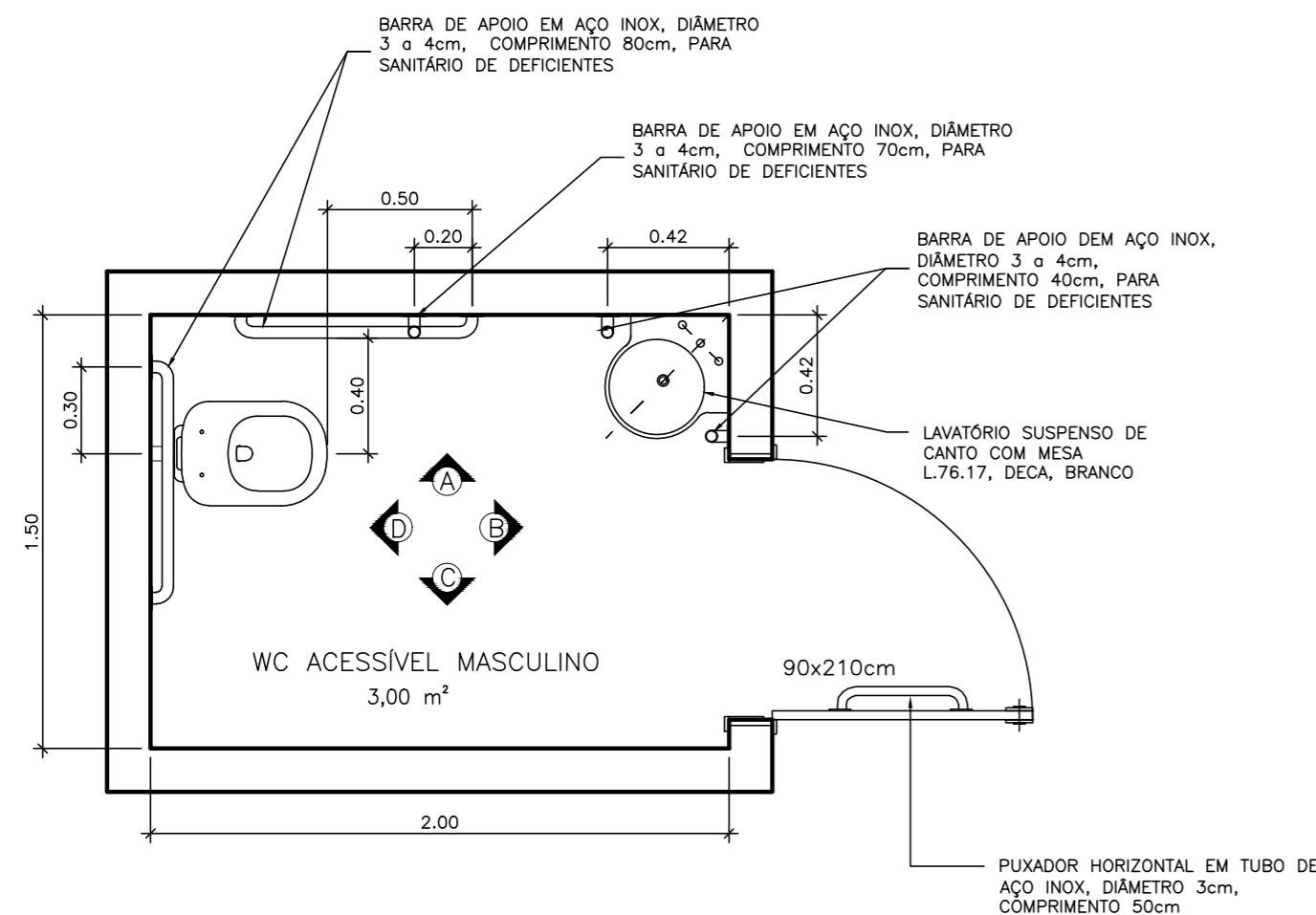
PLANTA BAIXA WC ACESS. MASC. ESCALA 1:25
