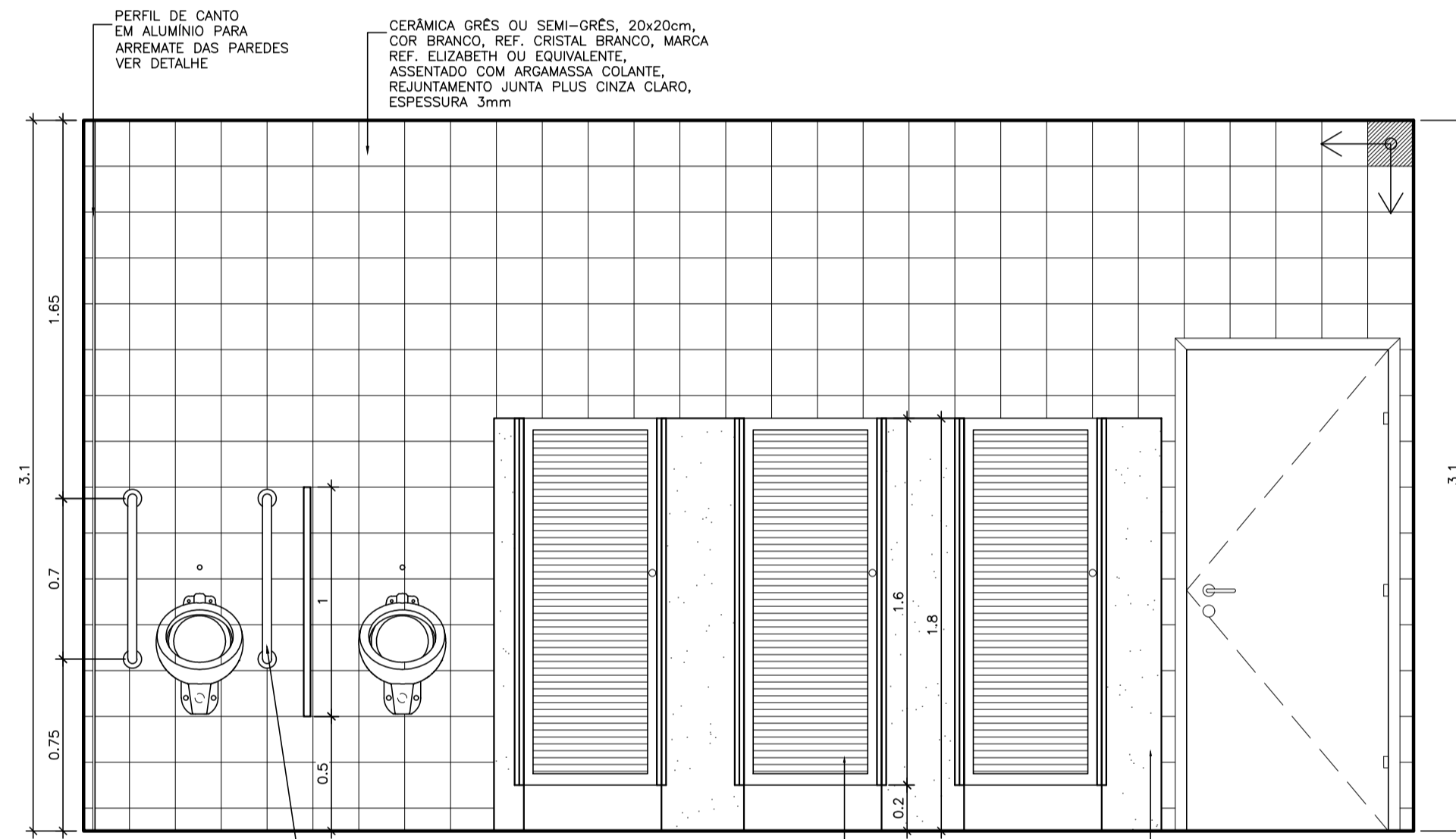
VISTA A ESCALA 1:25
