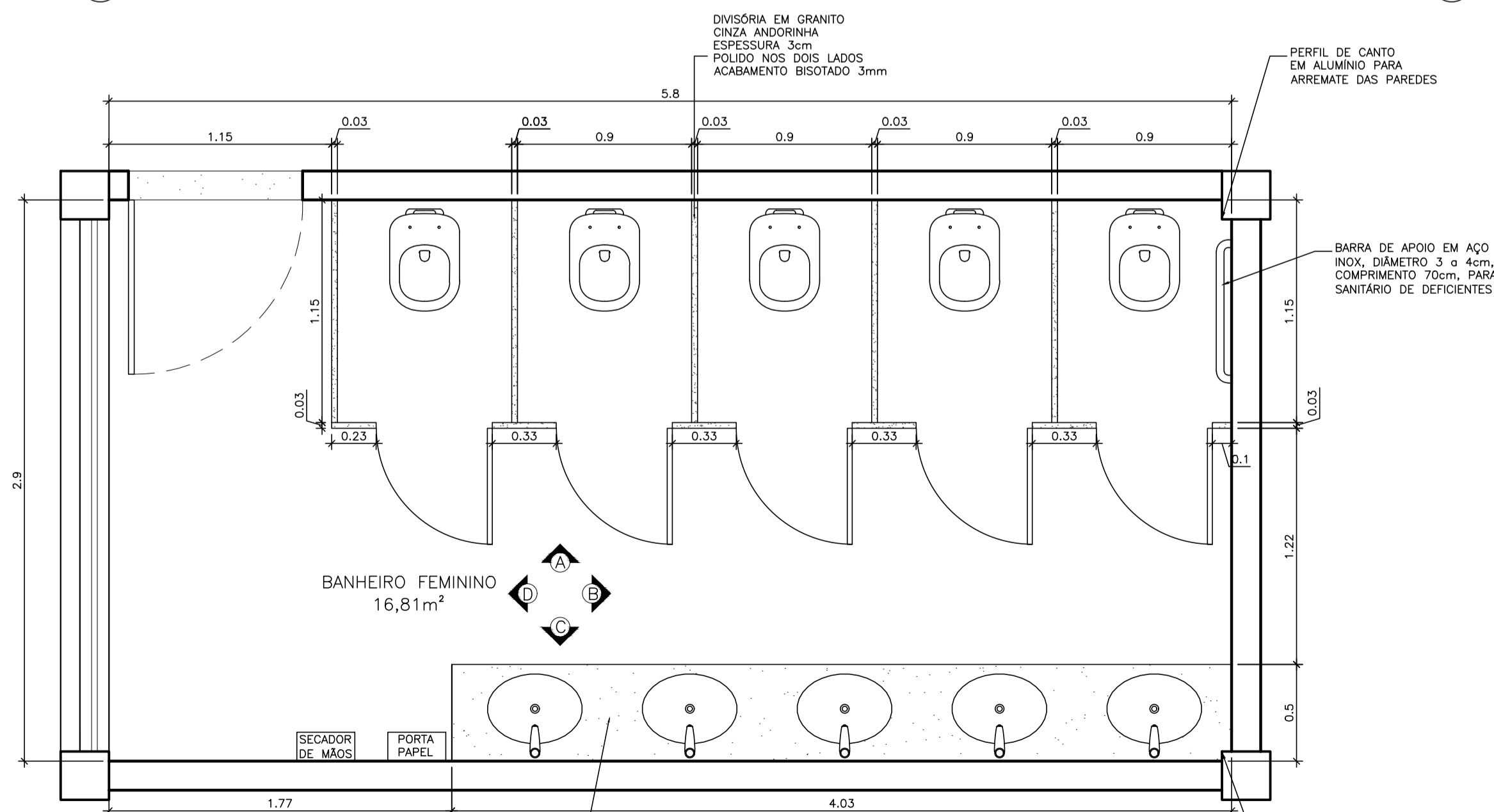
VISTA A ESCALA 1:25
