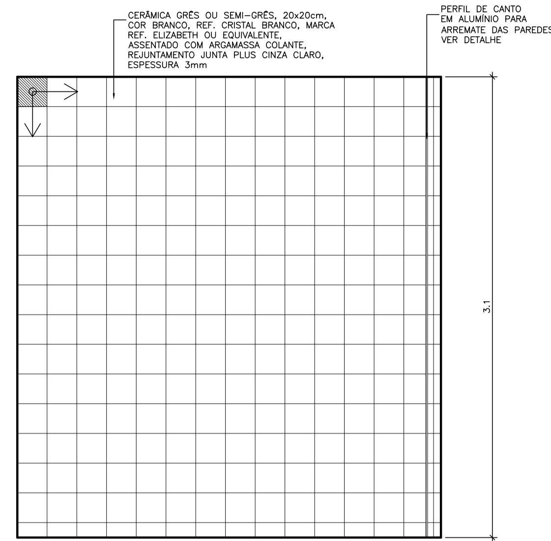
VISTA D ESCALA 1:25
