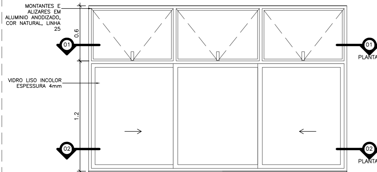
VISTA - J3
