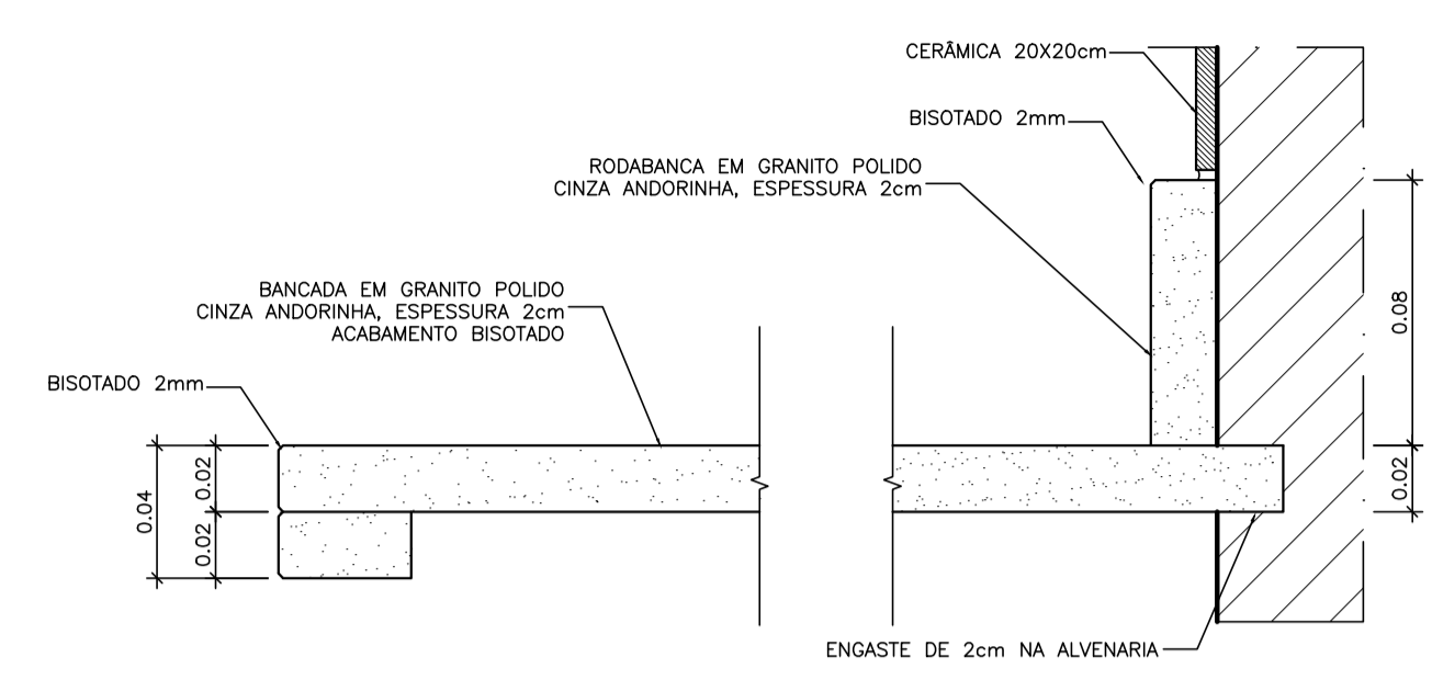
DETALHE BORDA E RODABANCA DA BANCADA ESCALA 1:2,5
