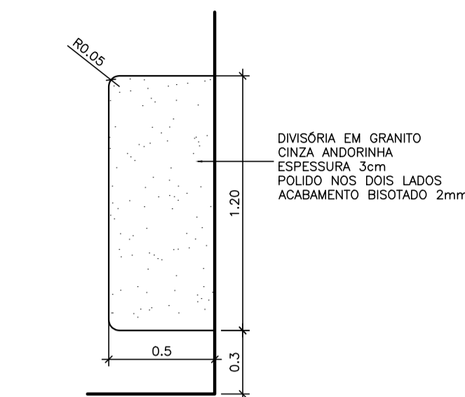
DET. DIVISÓRIA MICTÓRIOS ESCALA 1:25
