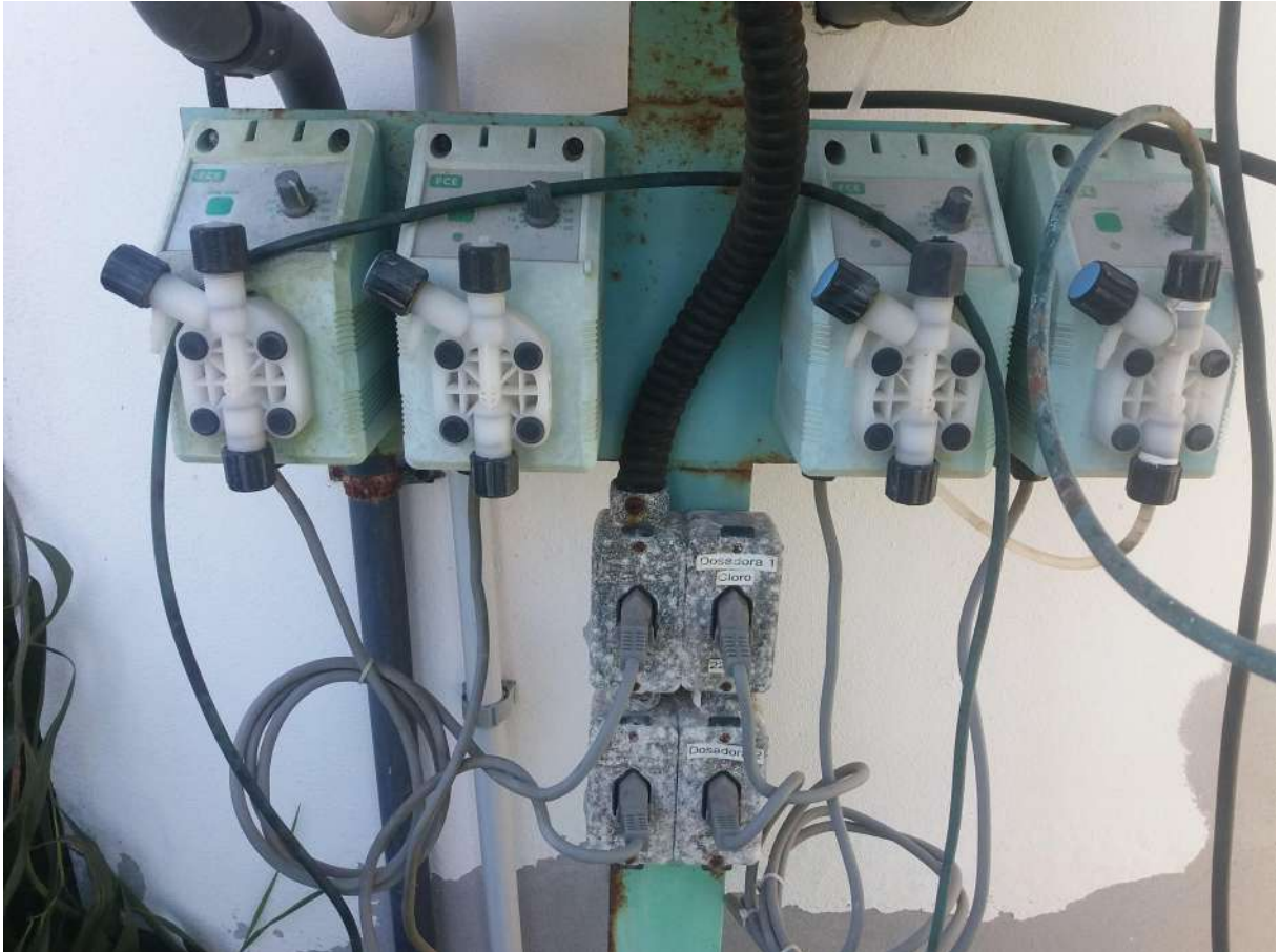
Foto 08: Substituição das mangueiras dos dosadores e verificação da funcionalidade
