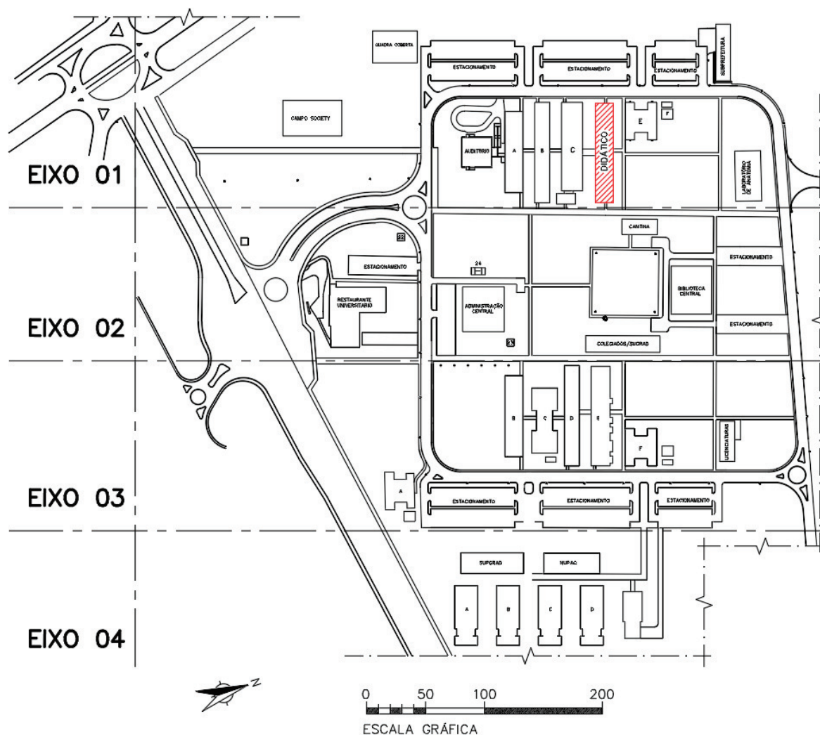
Figura 1: Planta de Situação da edificação a ser construída, destacada na cor vermelha.
